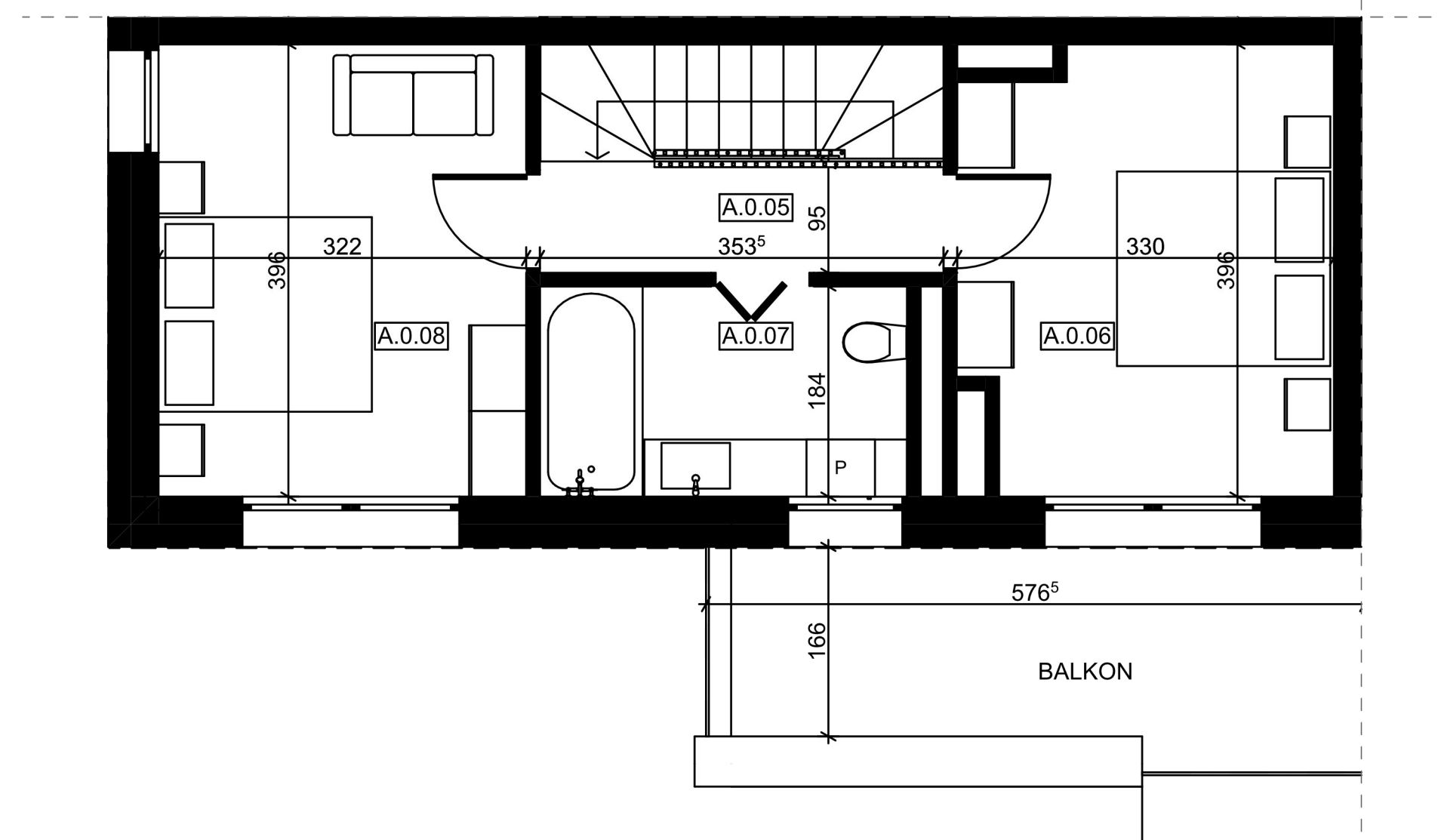
1. Piętro 1:50
