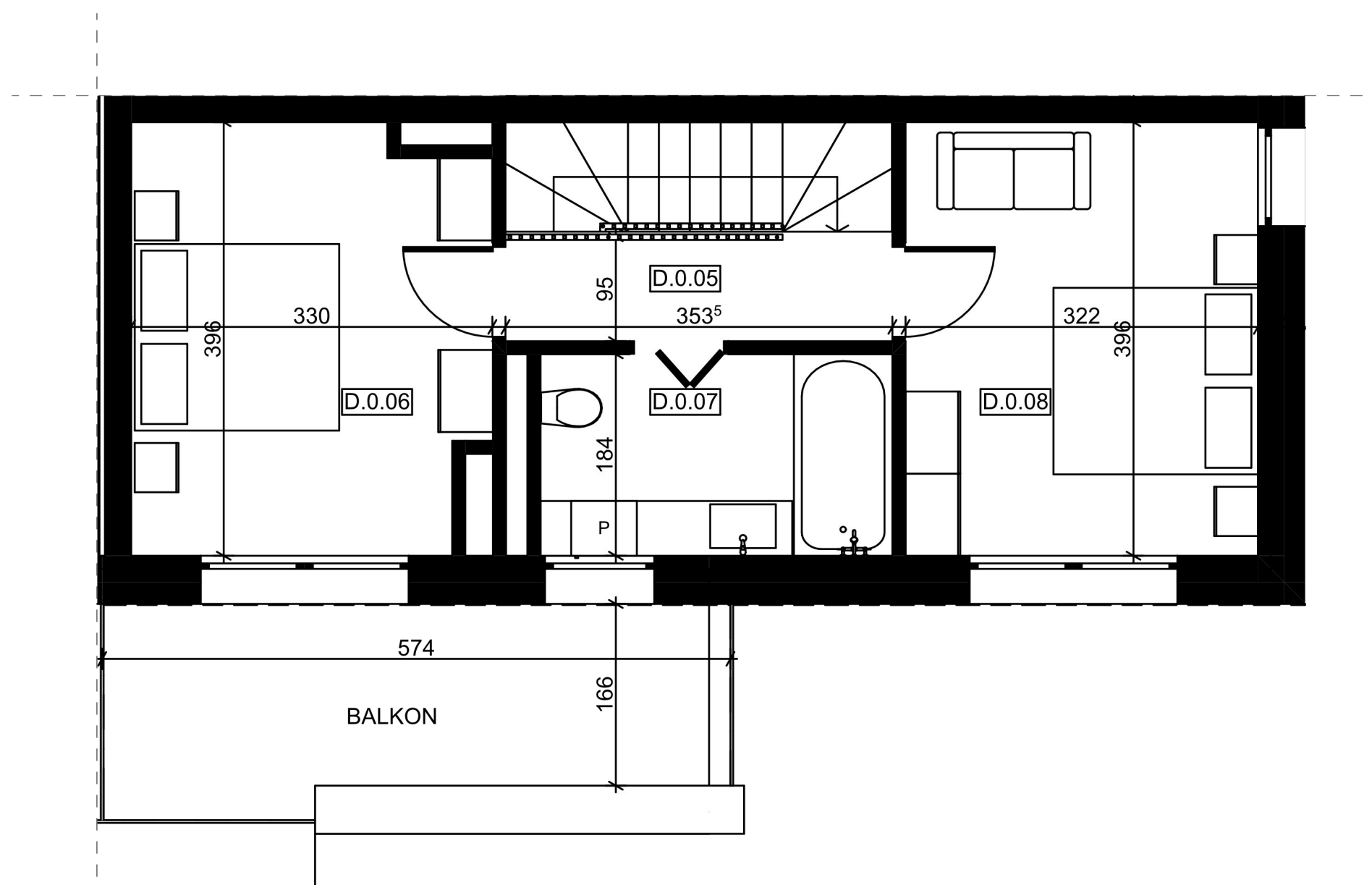
1. Piętro 1:50
